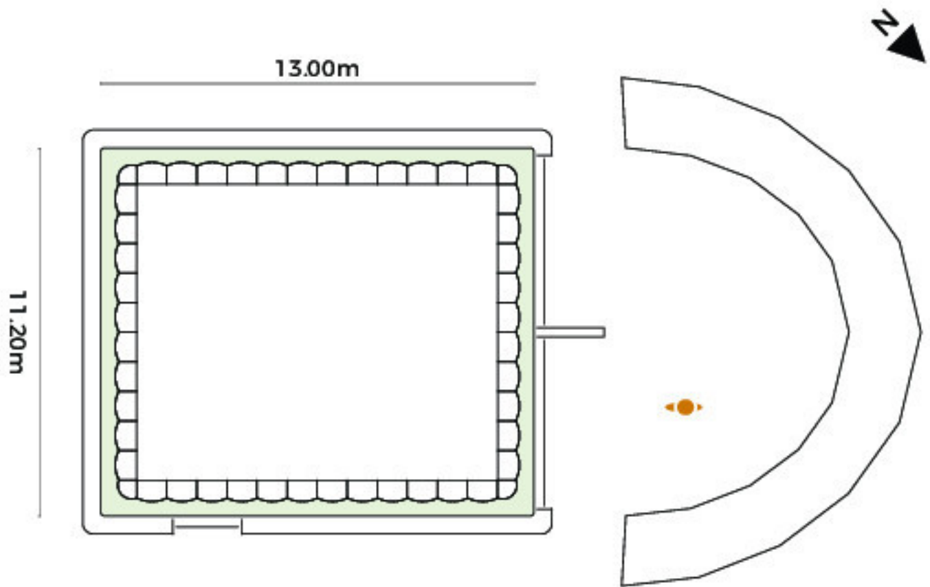
Ka`bah_Aufsicht_M1:300
